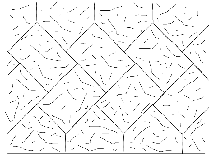
谷積標準立面図 S=1: 10
