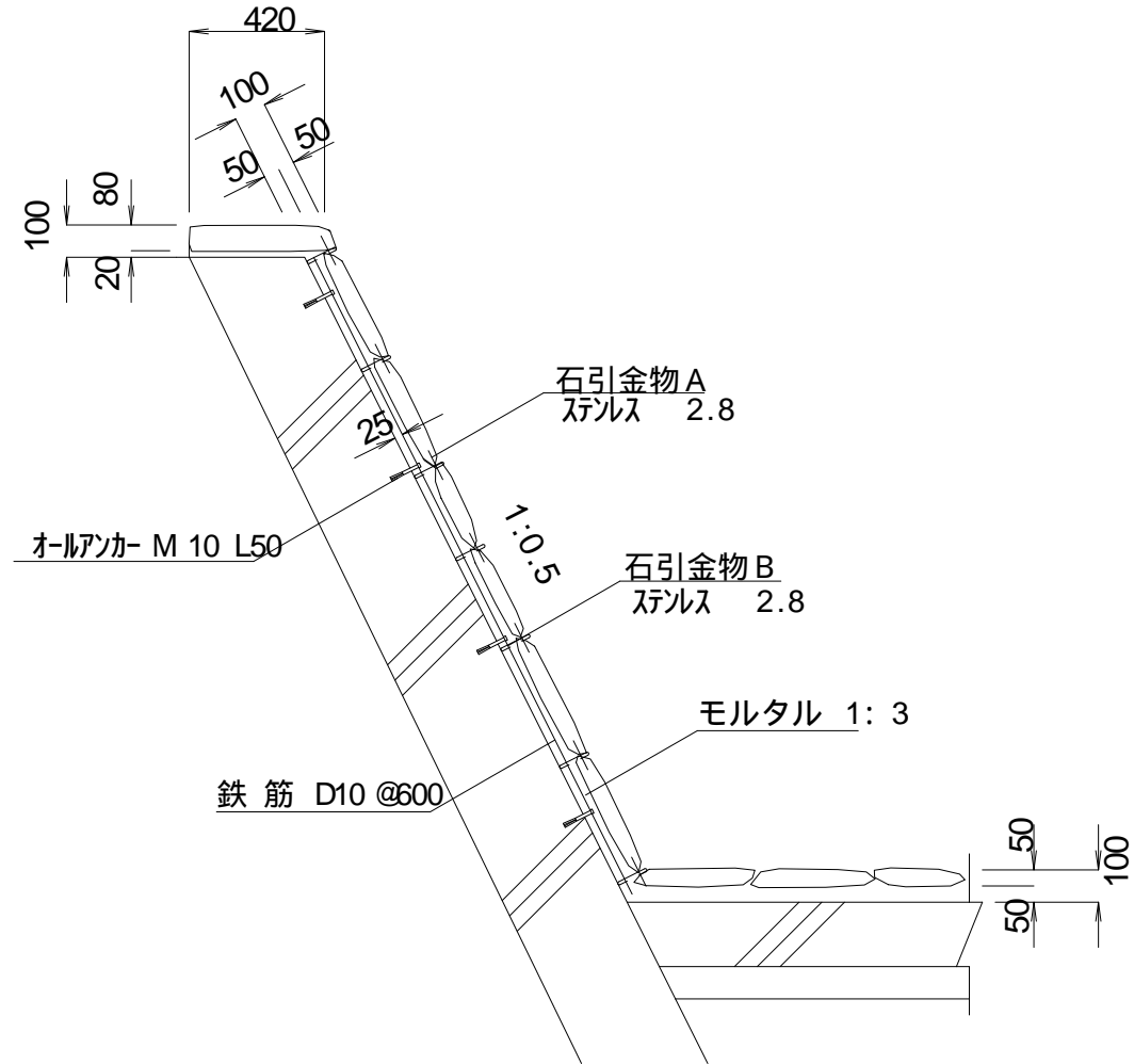
石張壁部及び底部断面図 S =1: 10
